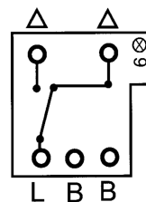
Koblingsskjema
